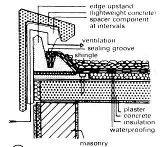
8 Concrete edge profile
